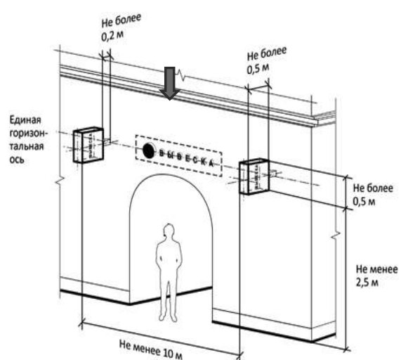
е) Максимальные параметры (размеры) консольных конструкций, размещаемых на фасадах объектов, являющихся объектами культурного наследия, выявленными объектами культурного наследия, не должны превышать 0,50 м - по высоте и 0,50 м - по ширине.
