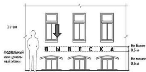
д) Вывески могут быть размещены над окнами подвального или цокольного этажа, но не ниже 0,60 м от уровня земли до нижнего края настенной конструкции. При этом вывеска не должна выступать от плоскости фасада более чем на 0,10 м
