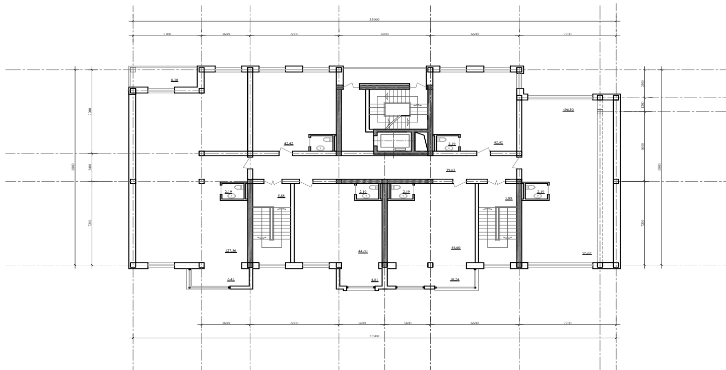
ПЛАН 2-го ЭТАЖА
