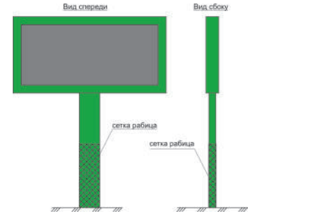
Рис.6 Эскиз опоры рекламной конструкции с закрепленной на ней сеткой рабицей
